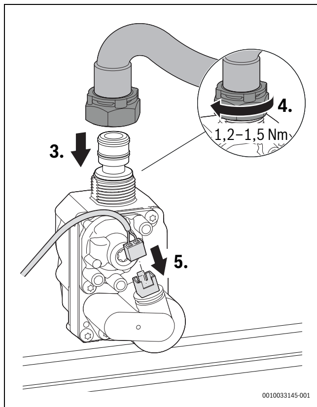
Мал. 78 Притягніть газовий шланг і штекер – Дотримуйтесь моменту затягування
