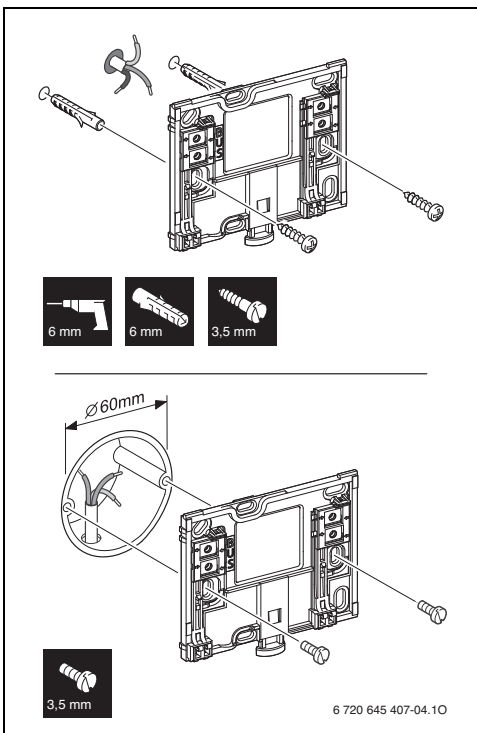
Мал. 3 Встановлення монтажної панелі
