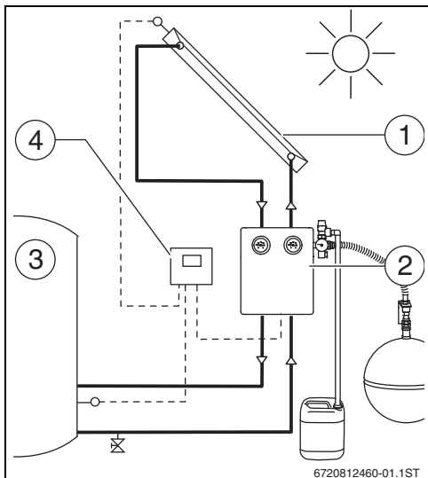
Рис. 3 Схема установки
