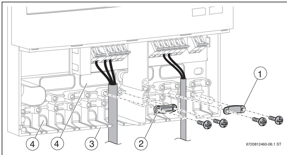
Мал. 7 Прокладання та кріплення кабелю
