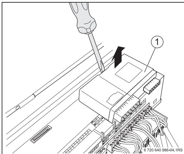
Мал. 10 Зняття функціонального модуля
