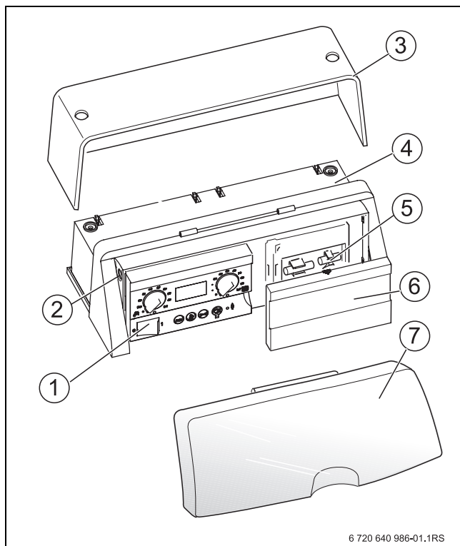
Мал. 1 Регулювальний прилад MC10
