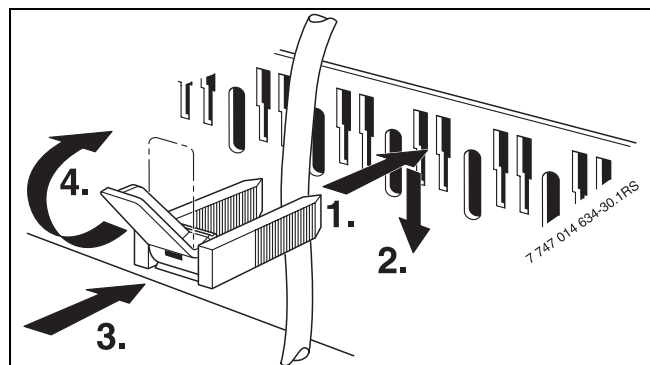
Мал. 4 Проведення кабелю та навантаження розтягування
