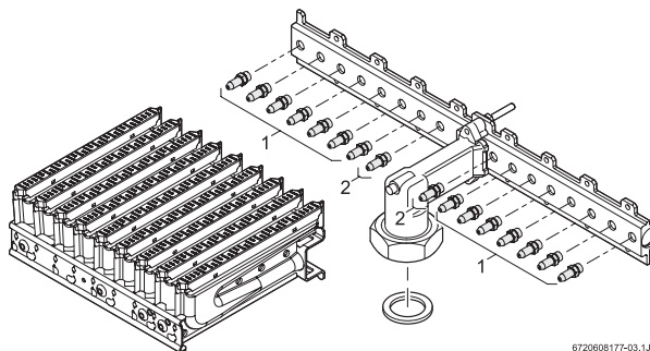
Рис. 3 Природний газ
