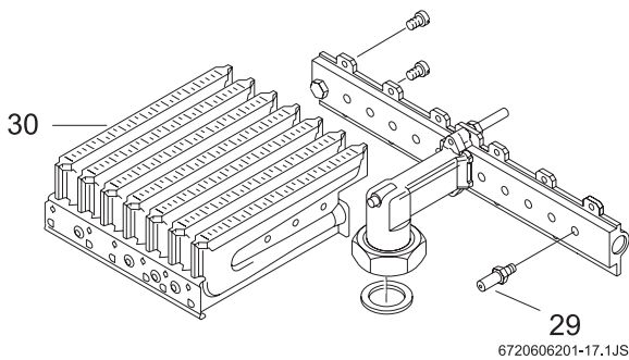
Рис. 4 Скраплений газ
