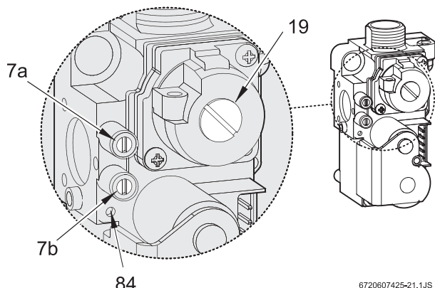
Рис. 6 Газова арматура
