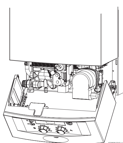
Рис. 5 Блок у сервісному положенні
