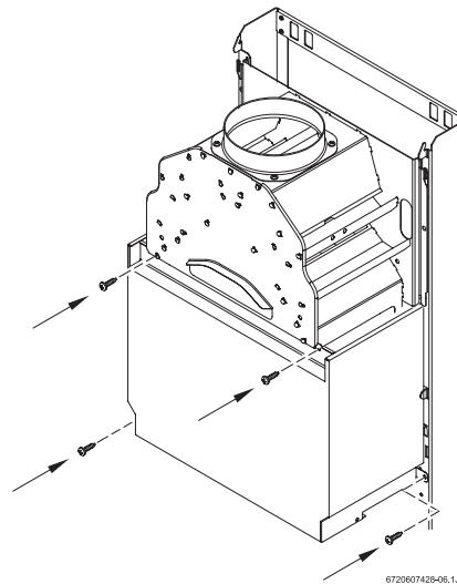
Рис. 1 Захисна кришка (ZS/ZW24-2-2DHKE)
